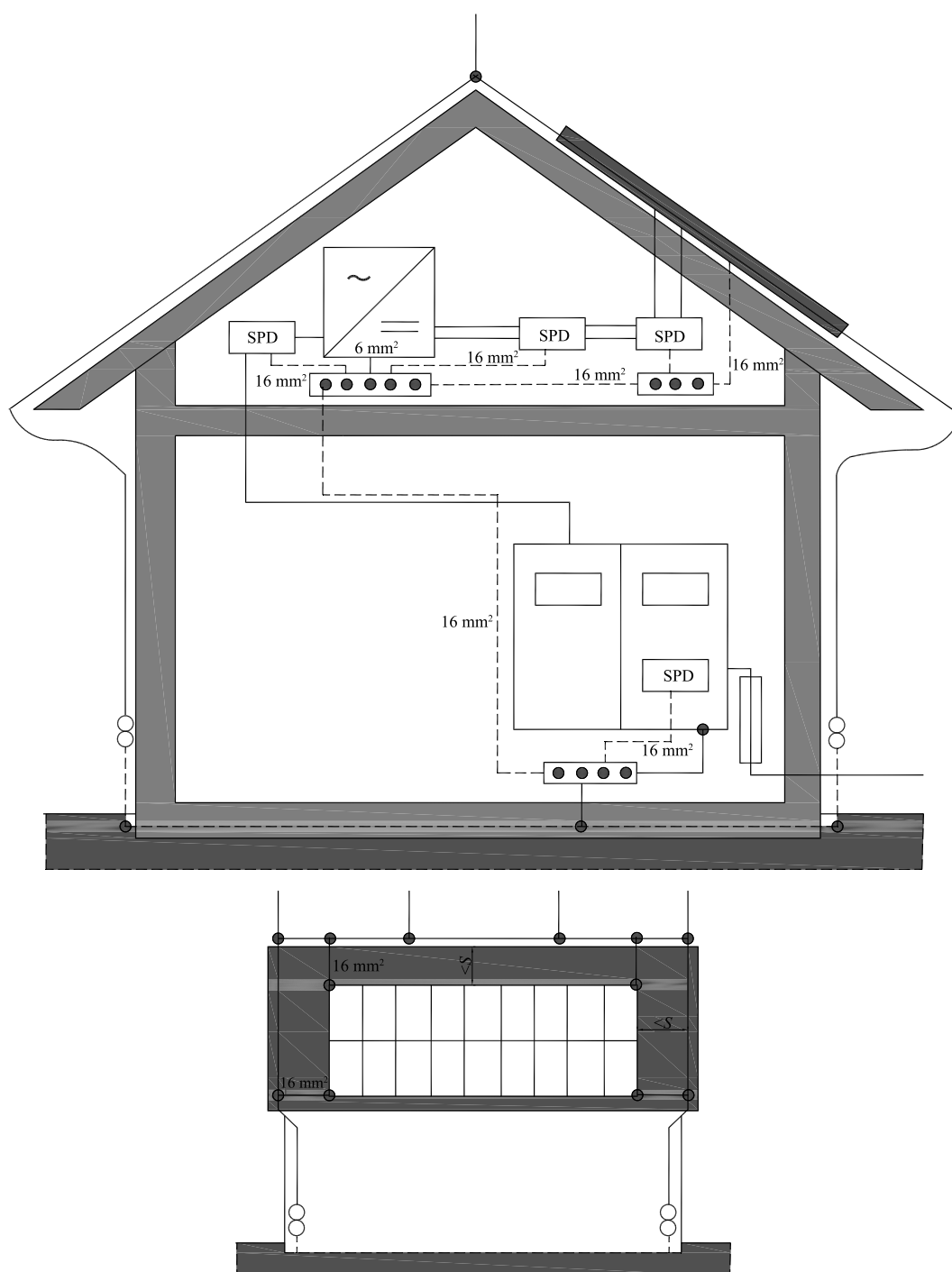
图 C.5 外部 LPS 不满足安全间隔距离的等电位连接导体的尺寸示例
